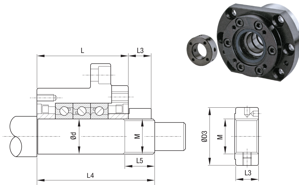
軸端尺寸
